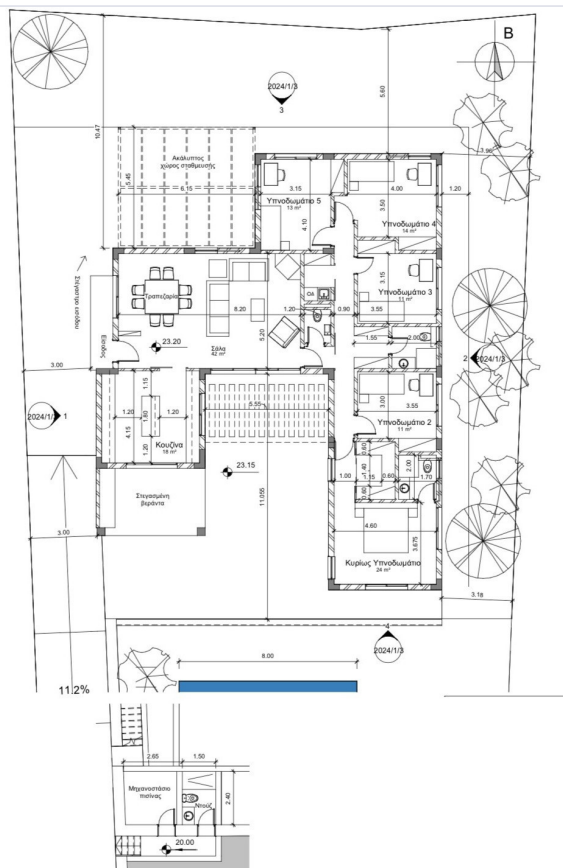
② Κάτοψη μηχανοστασίου παλινός 1:100
