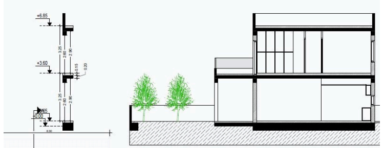
TOMH A-A
