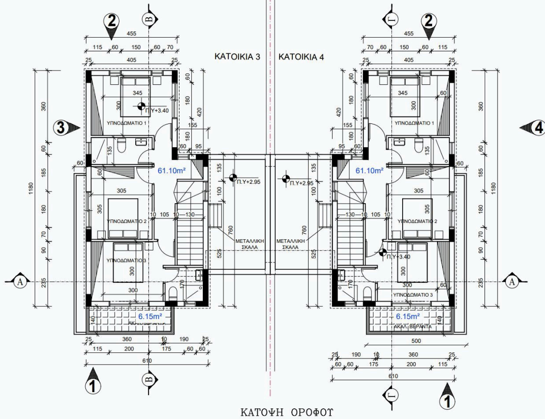
ΚΑΤΟΨΗ ΟΡΟΦΟΥ
