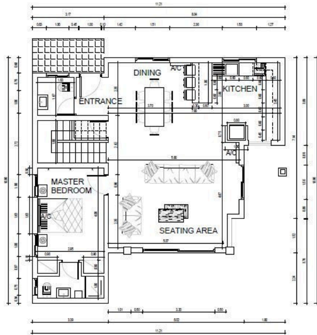
ΚΑΤΩΦΗ ΙΣΟΓΕΙΟΥ
