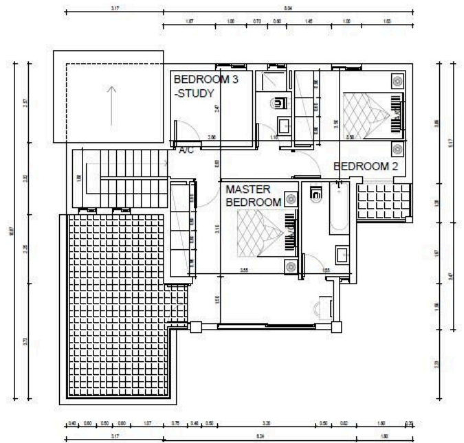
ΚΑΤΩΦΗ ΟΡΟΦΟΥ
