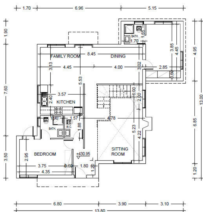
ΚΑΤΟΨΗ ΙΣΟΓΕΙΟΥ
