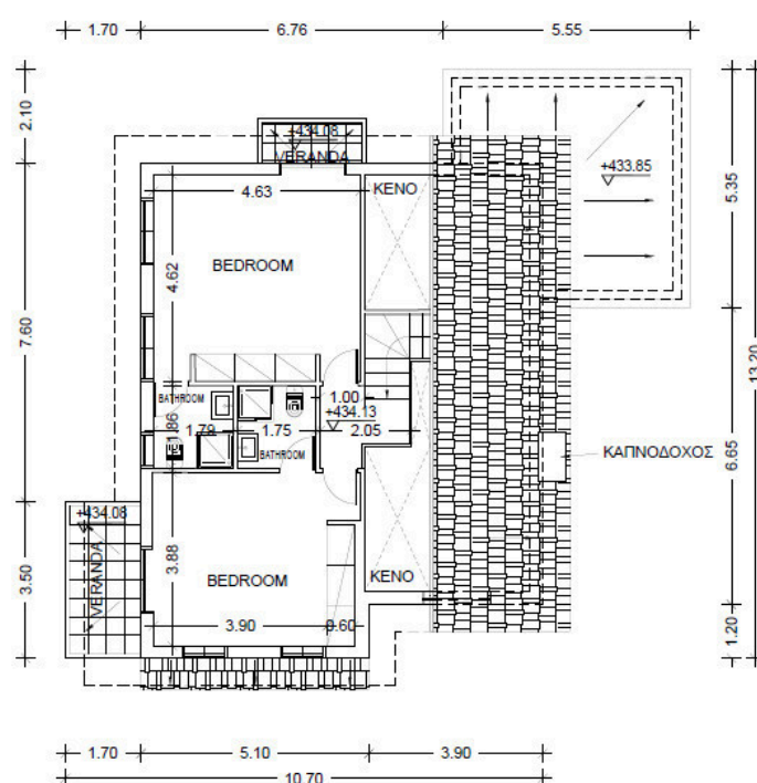
ΚΑΤΟΨΗ ΟΡΟΦΟΥ
