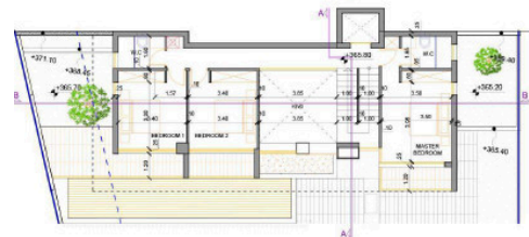
ΚΑΤΩΦΙ ΟΡΟΦΟΥ ΚΑ. 1:100
