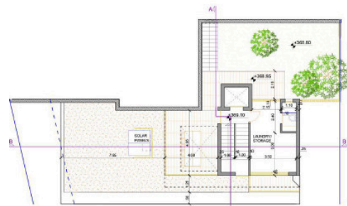
ΚΑΤΩΦΙ ΟΡΟΦΗΣ ΚΑ. 1:100
